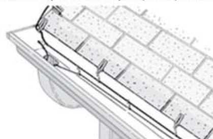
Figura 20b. Cable de ida y vuelta en canalones - solamente (canalones sin remaches internos)
